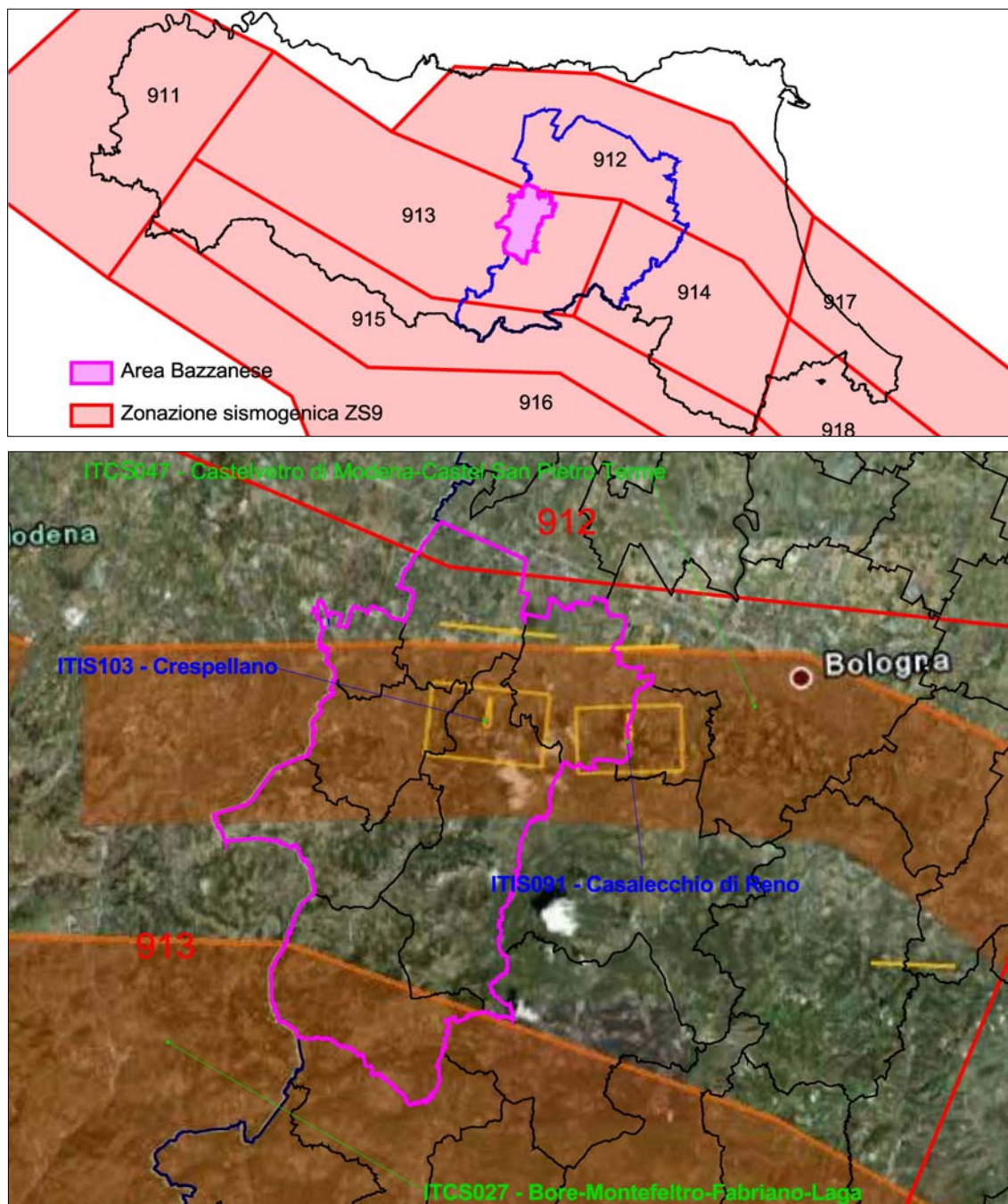
Fig. 2.7 Zonazione sismogenica ZS9 e distribuzione delle sorgenti sismogenetiche contenute in DISS 3.1 (foto aerea: Google Earth). Le sigle numeriche corrispondono alle "zone" sismogenetiche desunte dalla ZS9; le sigle ITCS corrispondono alle "zone" mentre le sigle ITIS corrispondono a "sorgenti" sismogenetiche della B/D DISS (versione aggiornata 3.1).
