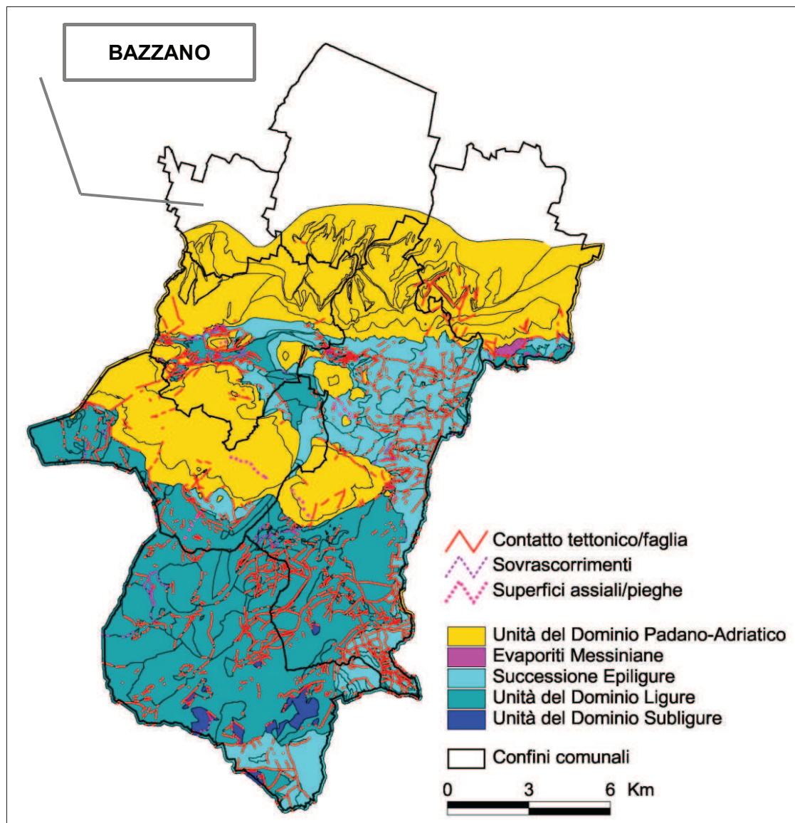
Figura 3.5 - Schema geo litologico del territorio collinare di Bazzano e degli altri Comuni dell'Area Bazzanese
