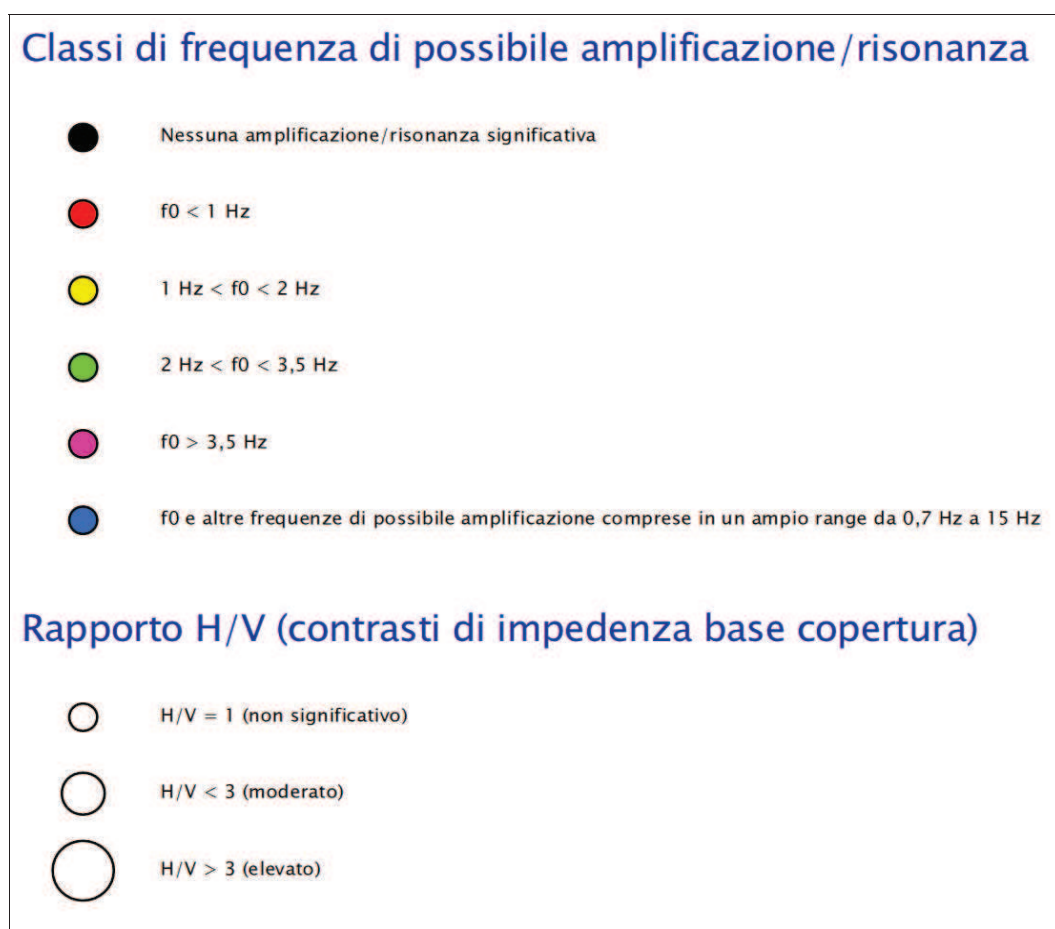
Figura 8.2 - Stralcio della legenda della <<Carta delle frequenze naturali dei terreni>> elaborata per lo studio di microzonazione sismica di Bazzano.
