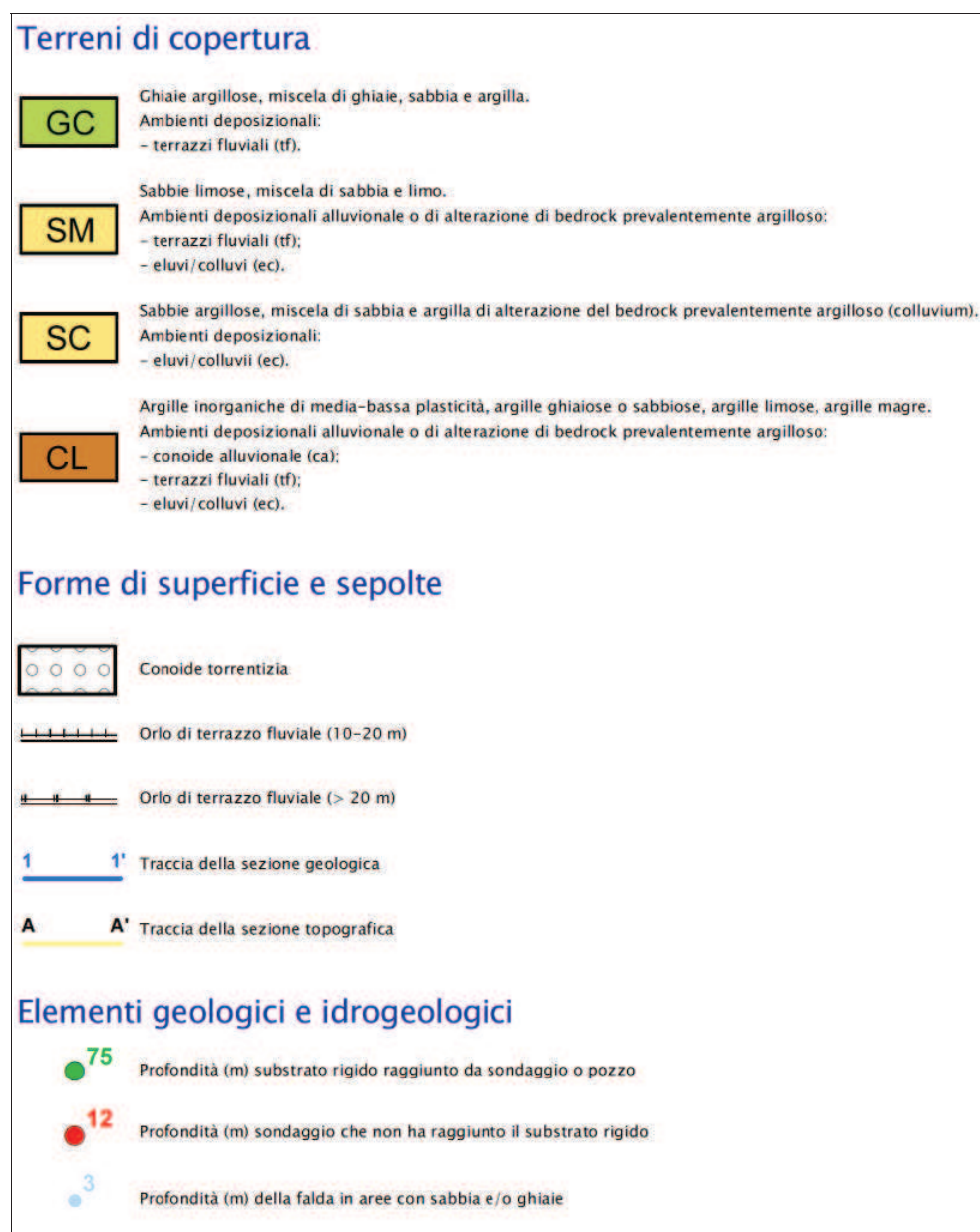
Figura 8.1 – Stralcio della legenda della <<Carta geologico-tecnica>> elaborata per lo studio di microzonazione sismica di Bazzano
