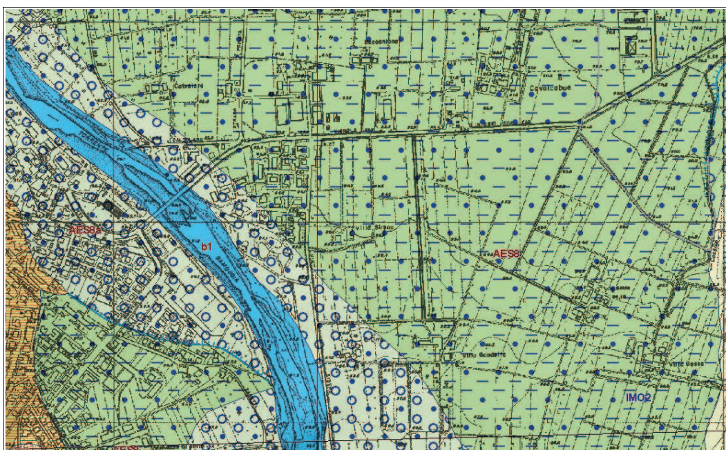
Figura 3.8 – Area Capoluogo (est): stralcio della Carta Geologica dell'Emilia-Romagna alla scala 1:10.000 , consultabile on line nel sito del Servizio geologico Sismico e dei Suoli RER.
