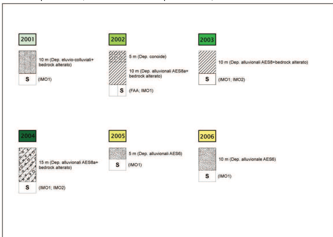
Figura 8.3 - Colonne stratigrafiche rappresentative delle microzone omogenee 2001-2002-2003-2004-2005-2006.
