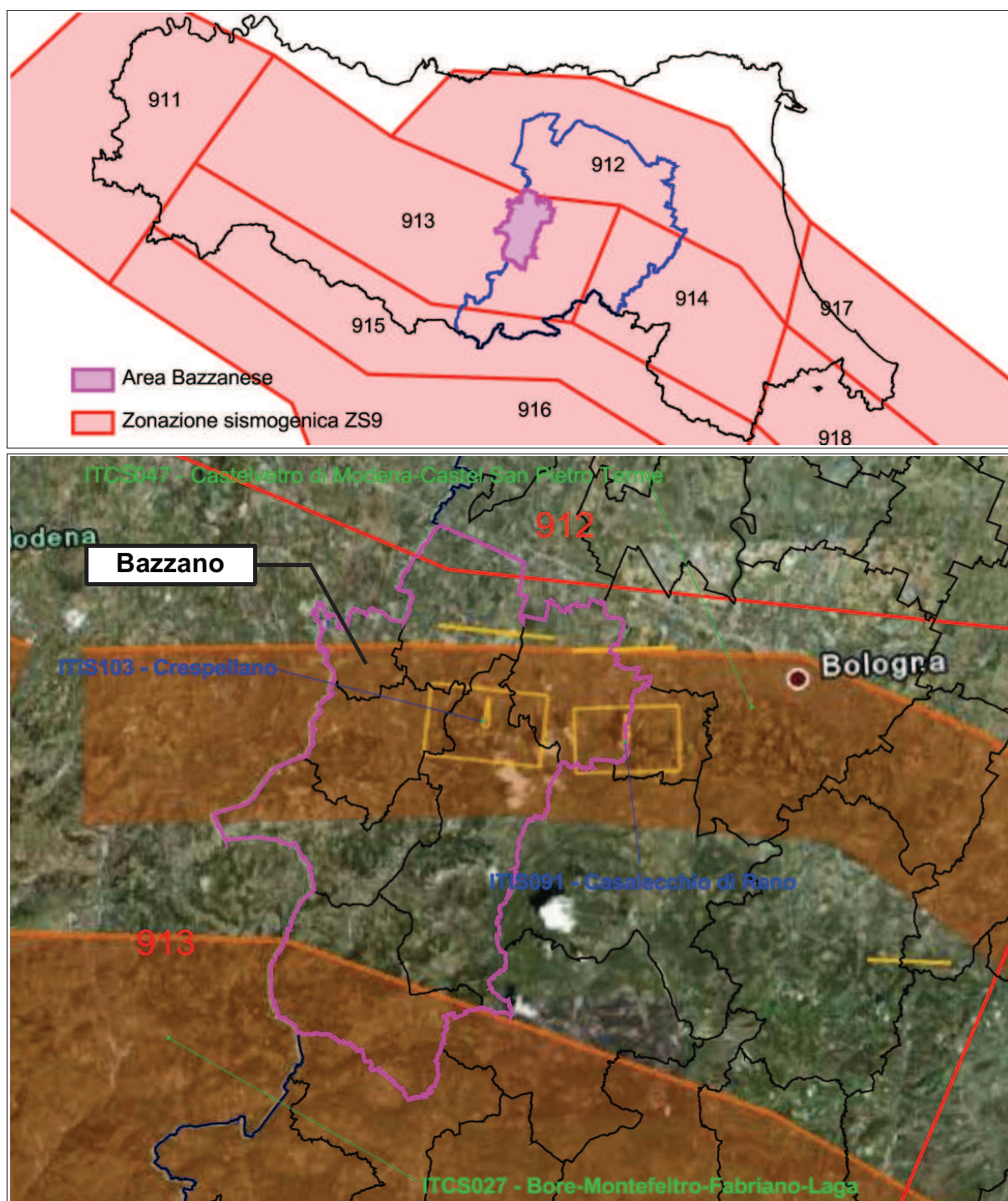
Figura 2.3 – Zonazione sismogenetica ZS9 e distribuzione delle sorgenti sismogenetiche contenute nel database DISS (versione aggiornata 3.1). Foto aerea: Google Earth. Nel database DISS le sigle ITCS corrispondono alle “zone” mentre le sigle ITIS corrispondono alle “sorgenti” sismogenetiche.
