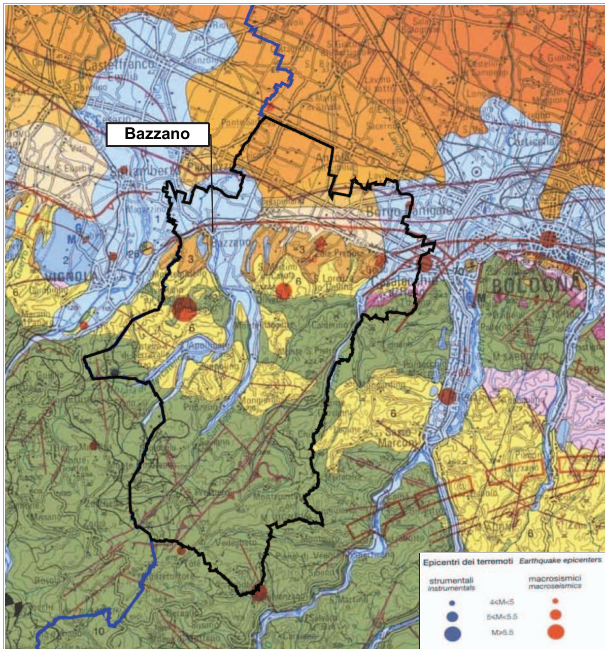
Figura 2.1- Sovrapposizione del territorio dei Comuni dell'Area Bazzanese (comprende anche il territorio di Bazzano) con la Carta Sismotettonica della Regione Emilia-Romagna (2004). Si riporta uno stralcio della legenda relativamente alla classificazione degli ipocentri dei terremoti strumentali di M_w > 4 e l'epicentro dei più significativi effetti macrosismici. La fonte regionale degli eventi sismici riportati è il catalogo parametrico nazionale dei terremoti storici (CPTI, 1999).
