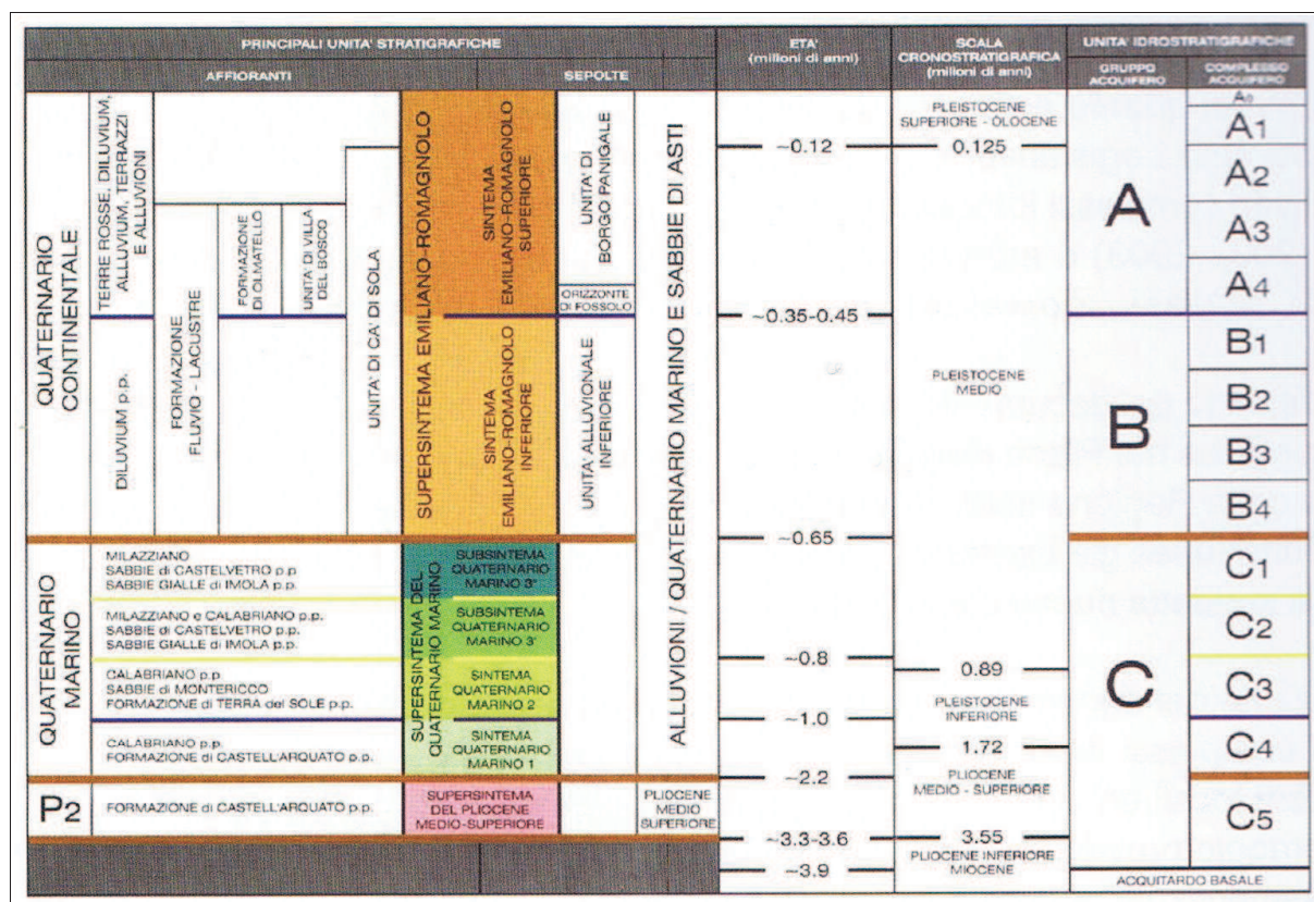
Figura 3.4 - Schema stratigrafico del margine appenninico e della pianura emiliano-romagnola (da: Regione Emilia-Romagna & ENI-AGIP, 1998, modif.). Sono evidenziati anche i rapporti tra unità deposizionali di pianura e i principali acquiferi.
