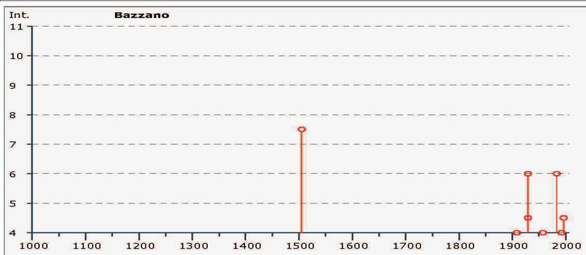
Figura 2.4 - Distribuzione dei terremoti significativi per il Comune di Bazzano e macrointensità stimata (fonte: INGV - Database Macrosismico Italiano 2011).
