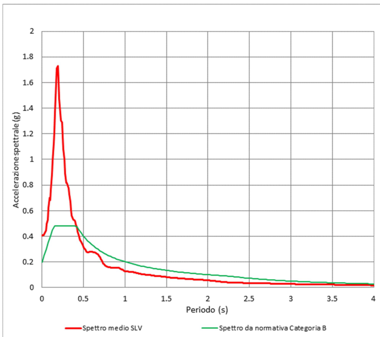
Figura 5-17 - Spettro medio di risposta in accelerazione per la verticale "Via Pontecchio", confrontato con lo spettro semplificato da normativa per la categoria di sottosuolo B
