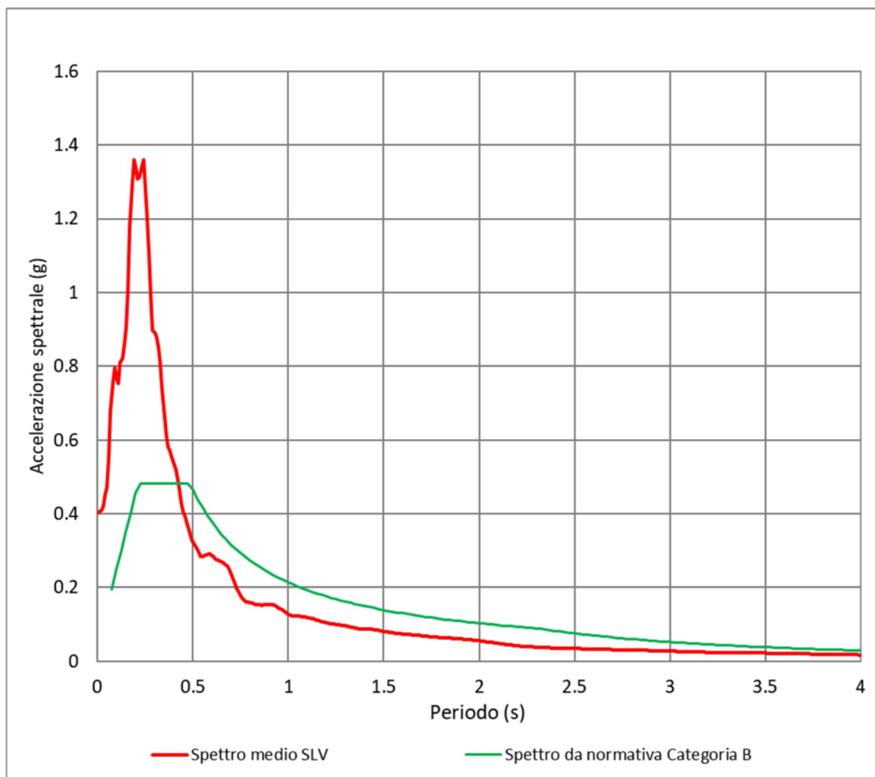
Figura 5-22 - Spettro medio di risposta in accelerazione per la verticale "Parco pubblico Via Achillini", confrontato con lo spettro semplificato da normativa per la categoria di sottosuolo B
