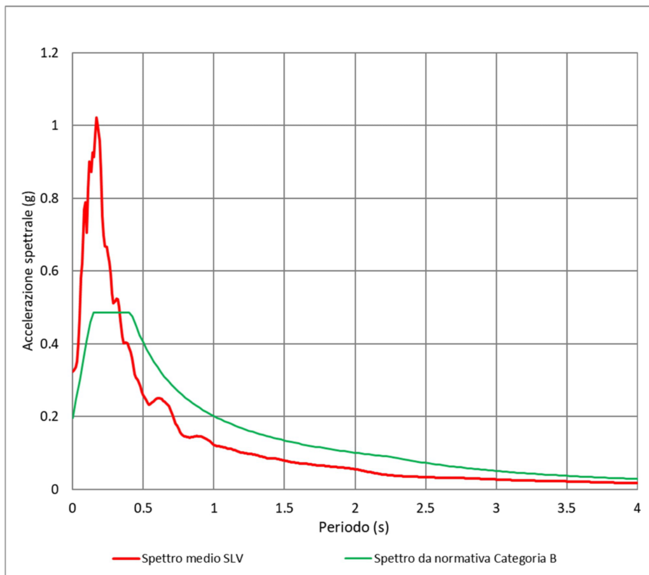
Figura 5-20 - Spettro medio di risposta in accelerazione per la verticale "Istituto Professionale B. Ferrarini", confrontato con lo spettro semplificato da normativa per la categoria di sottosuolo B
