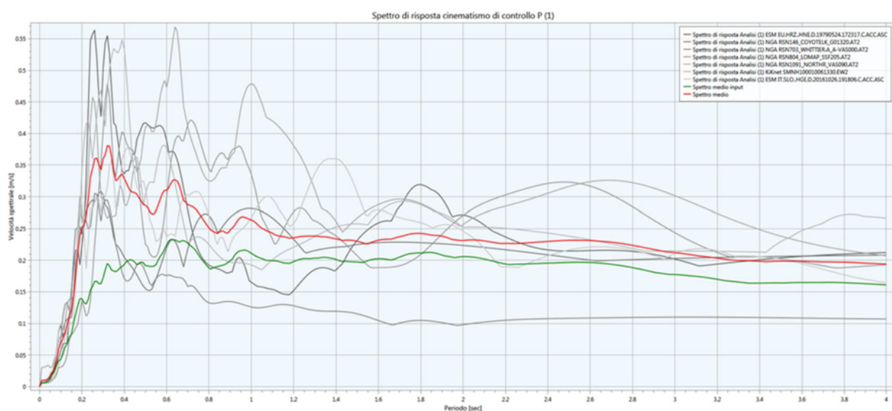
Figura 5-7 - Spettro elastico in velocità (in grigio gli spettri dei singoli accelerogrammi, in verde lo spettro medio di input, in rosso lo spettro medio di output)
