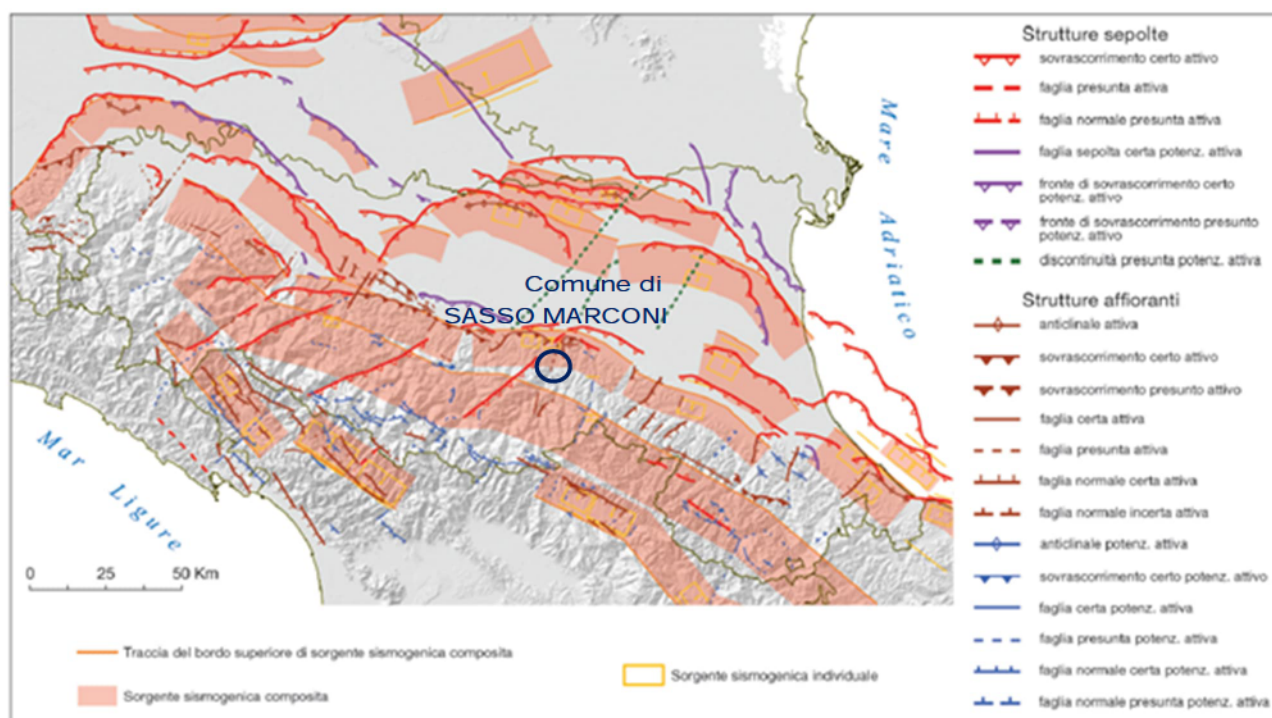
Figura 2-7 – Mappa di confronto tra le strutture tettoniche attive e potenzialmente attive riportate nella “Carta Sismotettonica della Regione Emilia Romagna ed aree limitrofe” e le zone sismogenetiche del DISS 3.2
