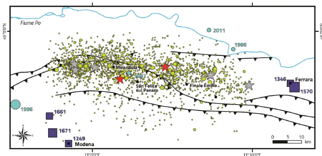
Figura 2-5 - Localizzazione della sequenza emiliana del 2012 e sismicità storica strumentale nell'area. (modificato da EMERGEO W.G., NHESS, 2013)
