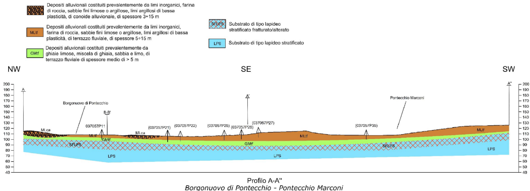
Figura 6-1 - Stralcio della sezione A-A'' (Borgonuovo di Pontecchio - Pontecchio Marconi)
