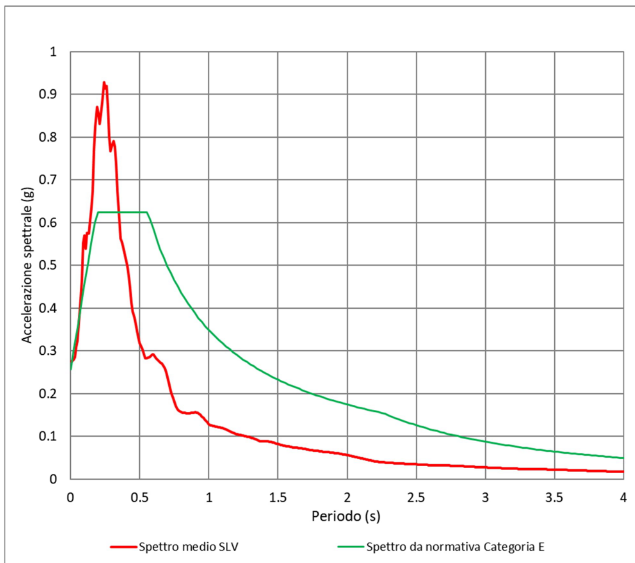
Figura 5-11 - Spettro medio di risposta in accelerazione per la verticale "Zona artigianale Pontecchio Marconi", confrontato con lo spettro semplificato da normativa per la categoria di sottosuolo E
