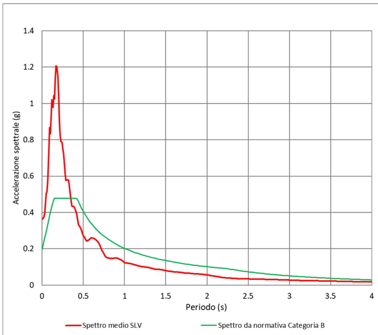
Figura 5-14 - Spettro medio di risposta in accelerazione per la verticale "Parco San Massimiliano Kolbe", confrontato con lo spettro semplificato da normativa per la categoria di sottosuolo B
