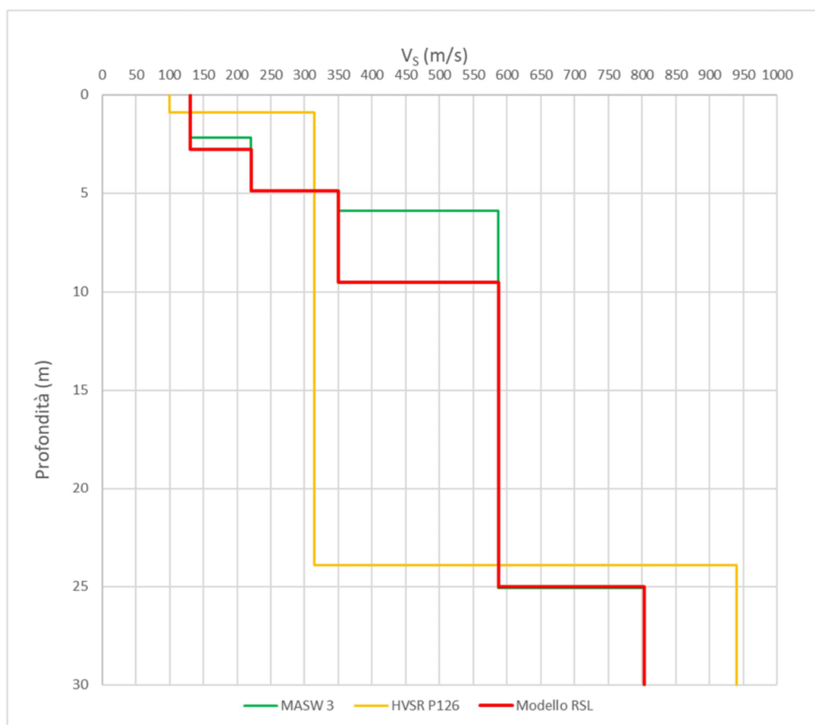
Figura 5-16 - Discretizzazione della V_s lungo la verticale "Via Pontecchio"
