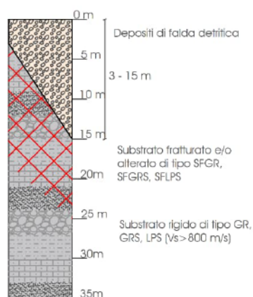
Figura 7-4 - Colonnine litostratigrafiche sintetiche, rappresentative delle microzone stabili suscettibili di amplificazioni locali
