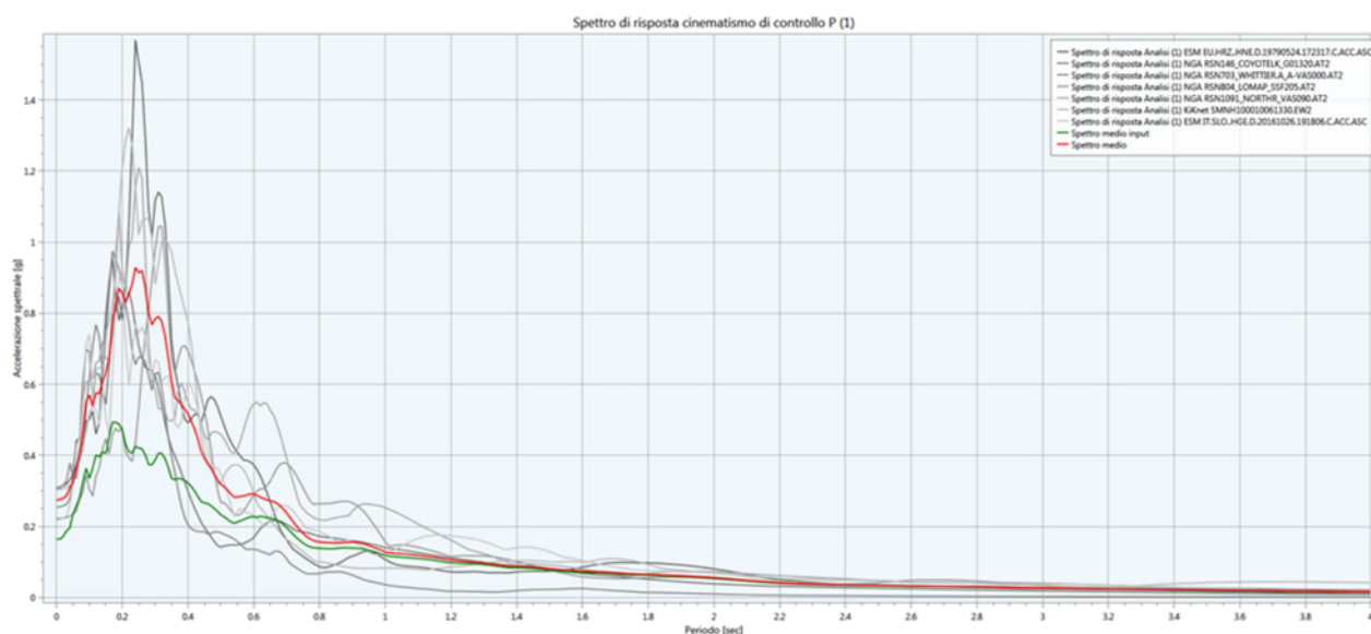
Figura 5-6 - Esempio di spettro elastico in accelerazione (in grigio gli spettri dei singoli accelerogrammi, in verde lo spettro medio di input, in rosso lo spettro medio di output)
