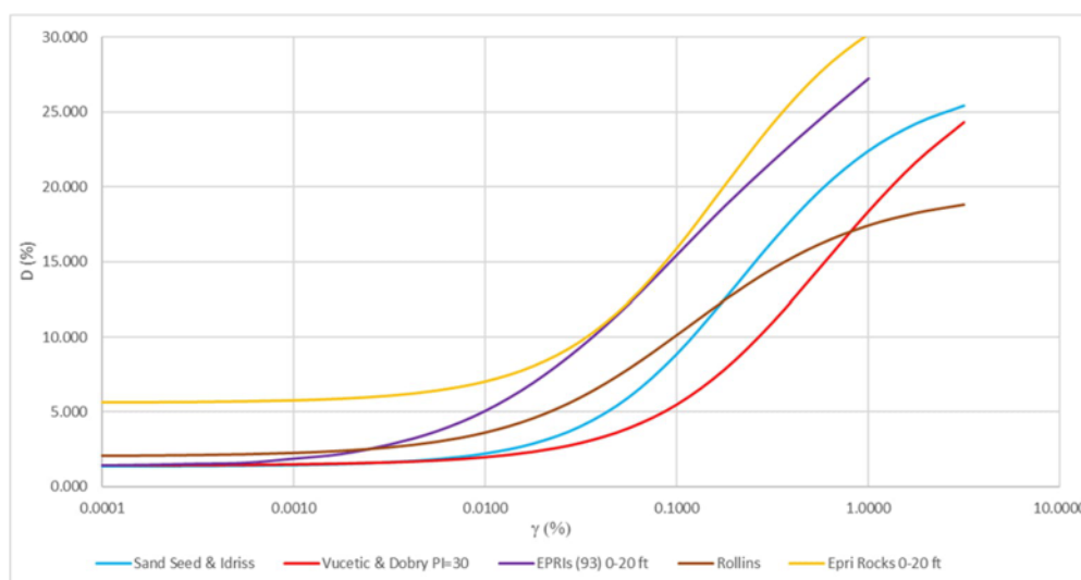
Figura 5-3 – Grafico delle curve di interpolazione D in funzione della deformazione
