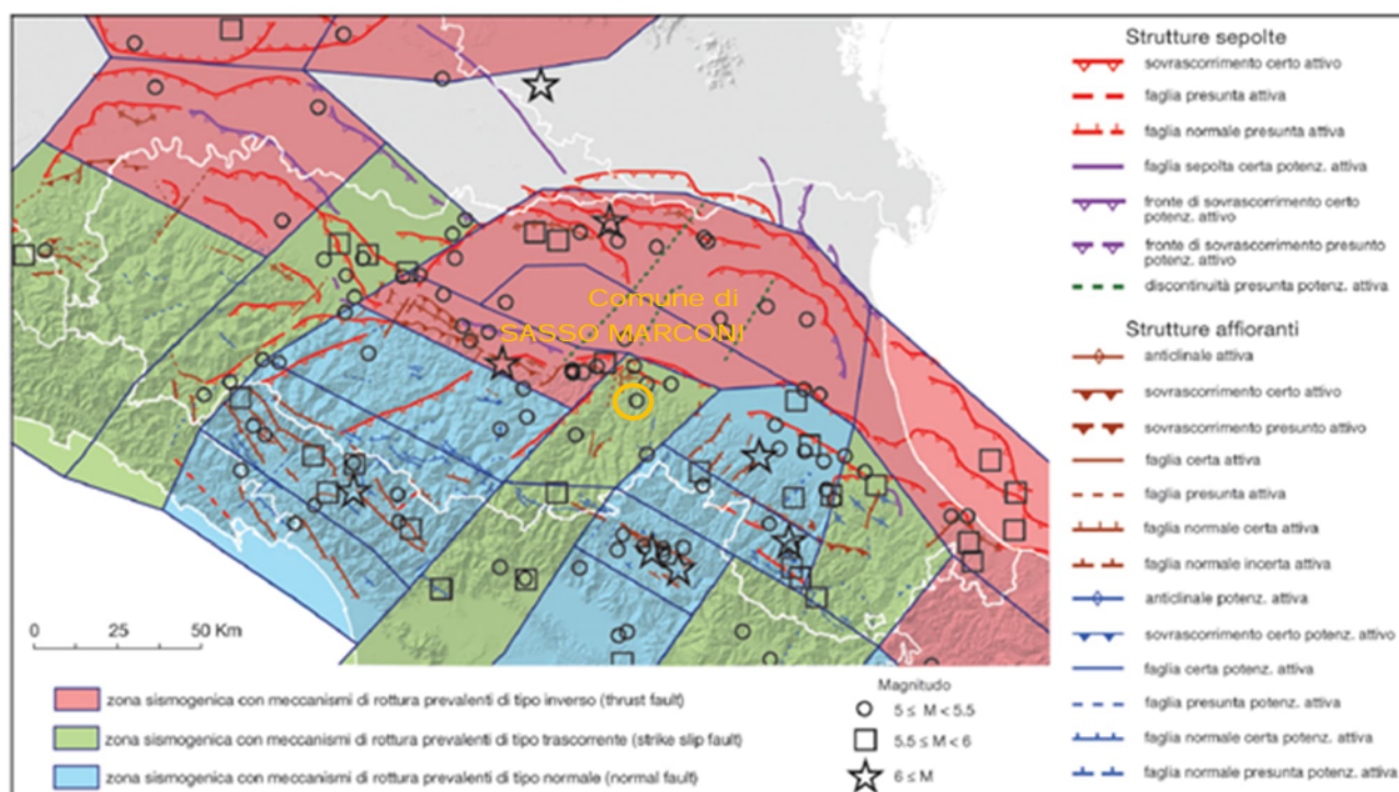
Figura 2-9 – Mappa di confronto tra le strutture attive e potenzialmente attive riconosciute e la zonazione sismogenetica proposta da Martelli et alii (2017)
