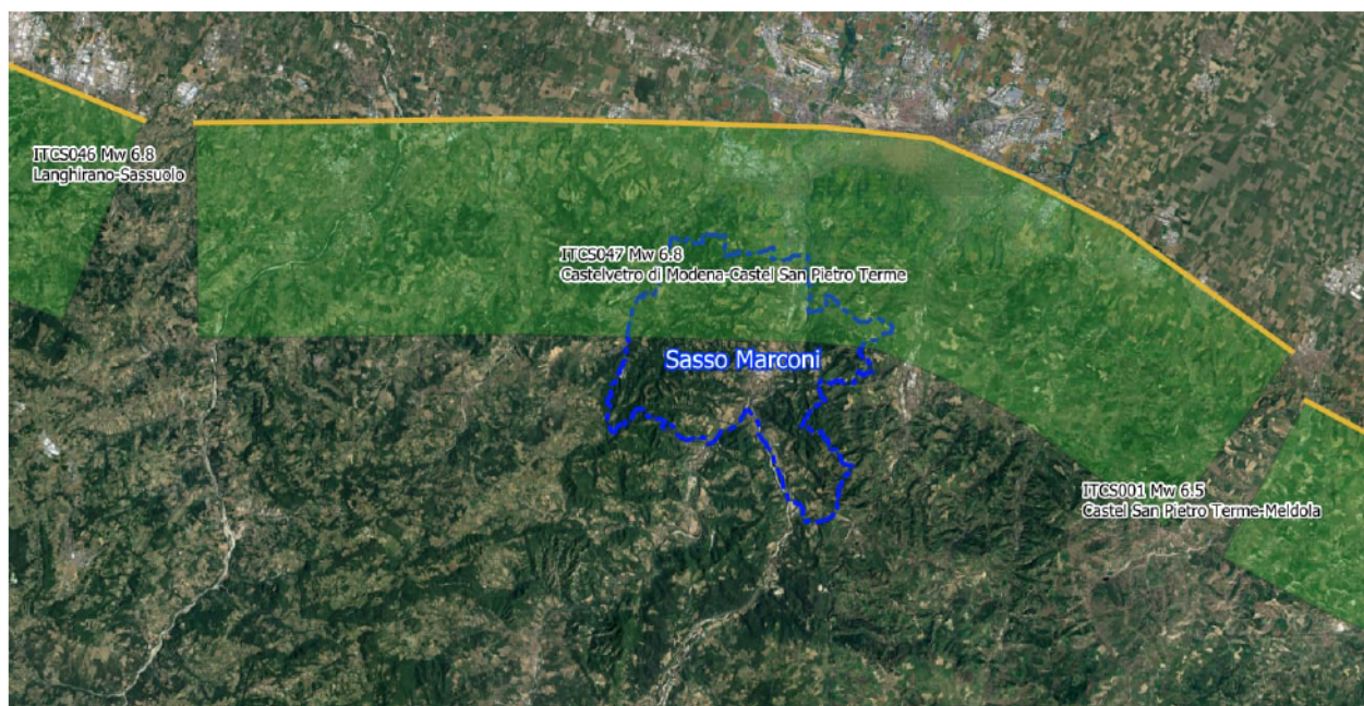
Figura 2-12 - Stralcio del DISS 3.3.0
